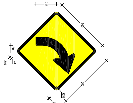
W1-3A(R) 600 x 600
